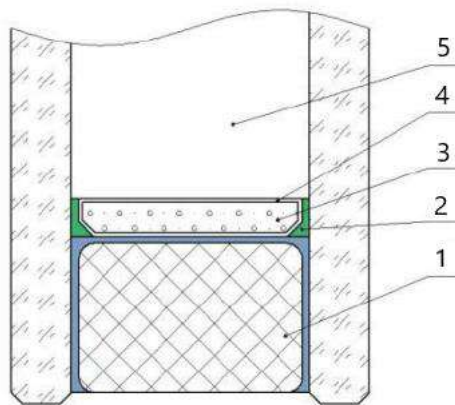
Рис. 2. Склопакет підвищеної жорсткості [6]: 1–підсилюючий контур (компонентний профіль), 2 – бутиловий герметик, 3 – абсорбент, 4 – дистанційна рамка, 5 – повітря або інертний газ.
