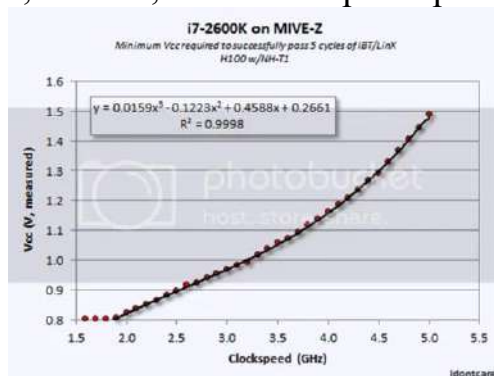
Рис. 7. Тести термоінтерфейсів
