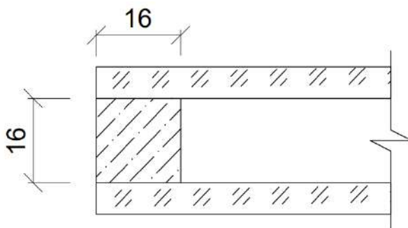
Рис. 3. Розрахунковий вузол склопакету
