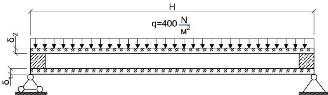
Рис. 4. Схема випробувань склопакета на навантаження
