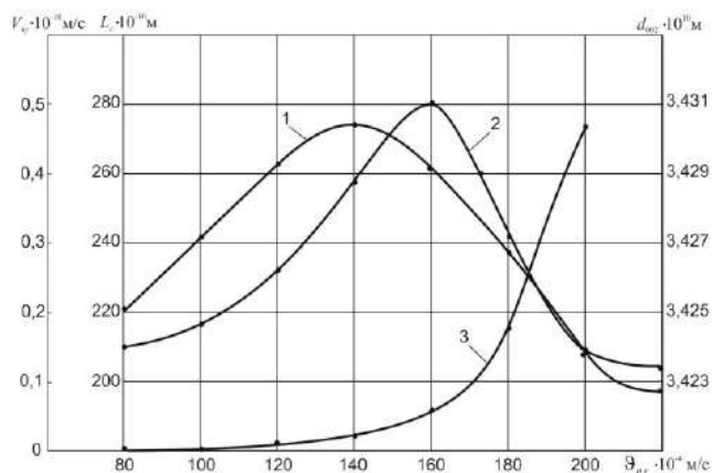
Рис. 2. Вплив швидкості потоку реакційних газів в реакторі Q_{p,г} на висоту кристалітів L_c (1), міжплощину відстань d_{002} (2) і швидкість осадження піролітичного графіту V_{ос} (3)
