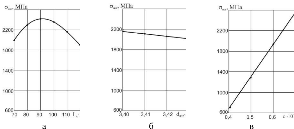
Рис. 1. Залежності межі міцності на вигин піролітичного графіту від висоти кристалітів (а) міжплощинної відстані (б) і мікроструктурної деформації (в)
